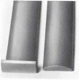
Abschluß-Schweißung
