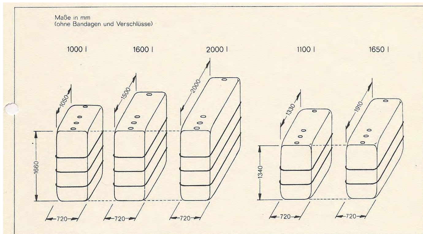
Batterie-Tanks
