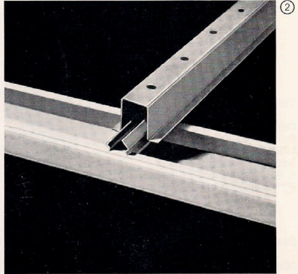
② Anschließend erfolgt das Einrasten der Klipps in die U-Schiene durch leichten Druck von unten.
