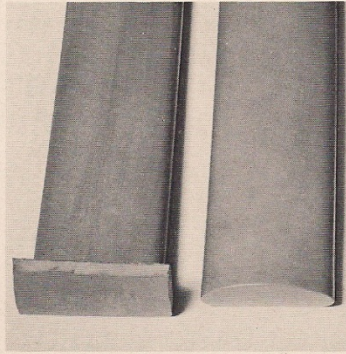
Abschluß-Schweißung
