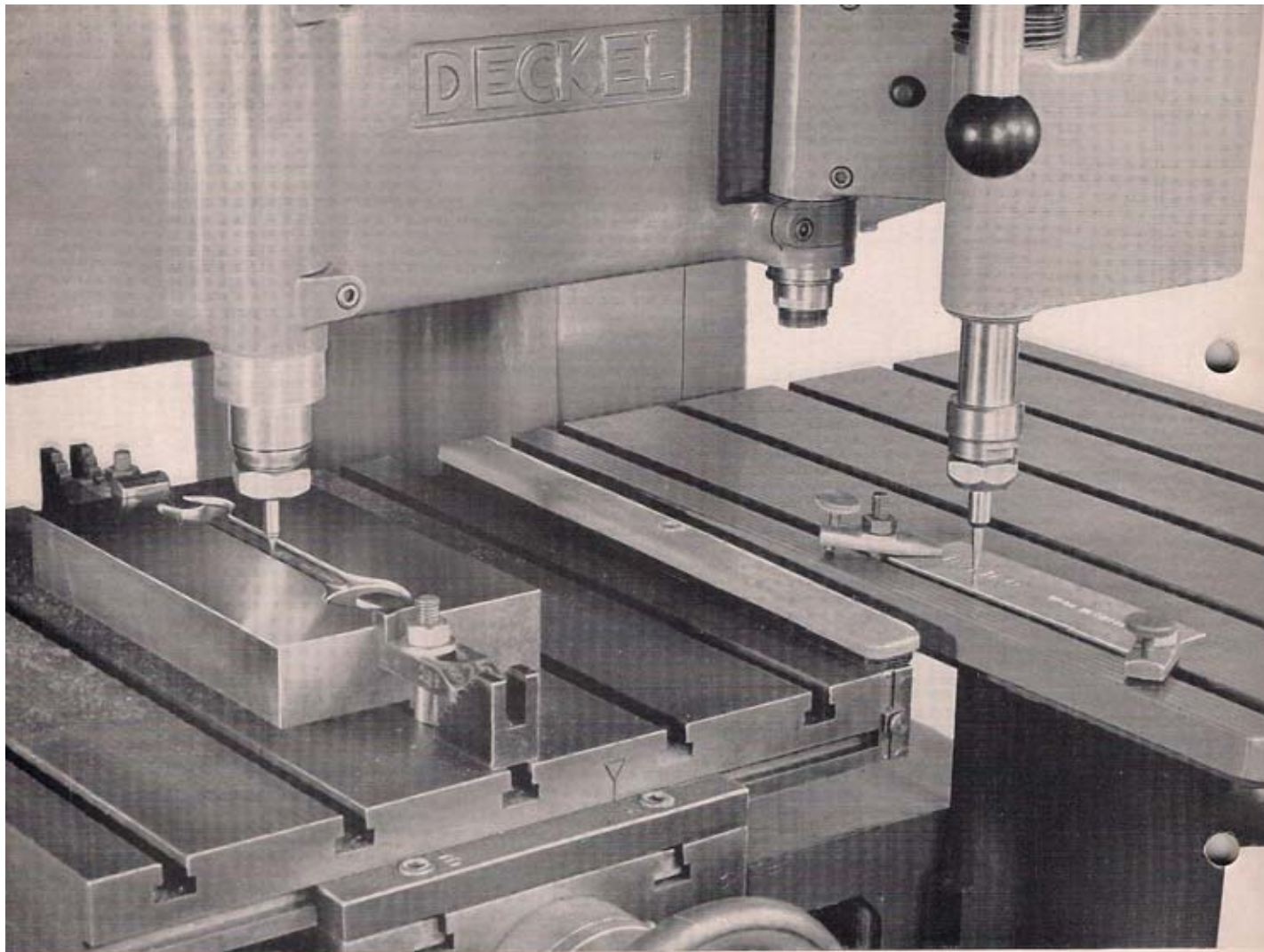
Arbeitsvorgang: Gravieren des Schriftzuges in das Trolon-Modell
