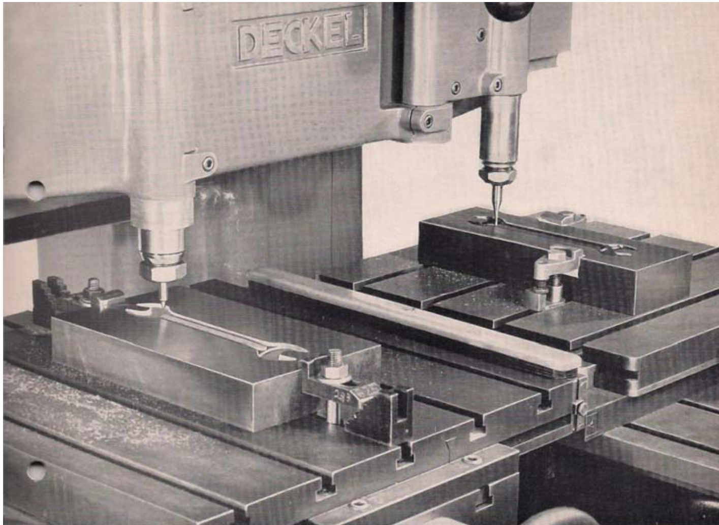
Arbeitsvorgang 2: links Stahlblock, rechts Trolon-Modell
