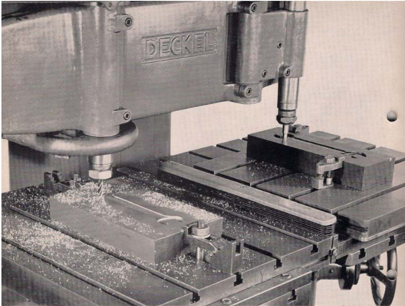
Arbeitsvorgang 1: links Stahlblock, rechts Trolon-Modell
