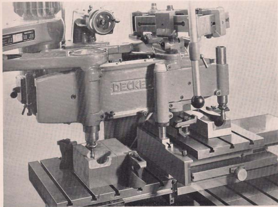
Spiegelbildfräsen in Trolon
