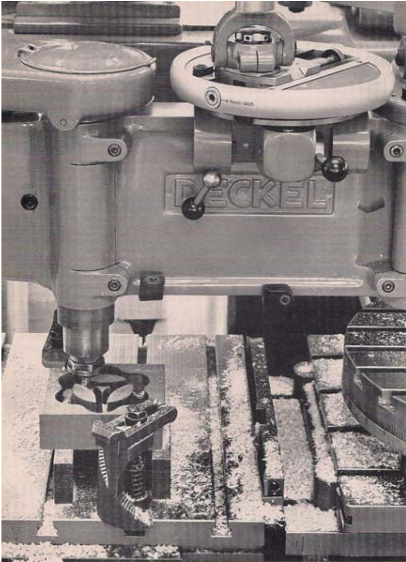
Ausarbeiten eines Speichenrades in Trolon
